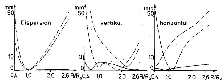
Fig.9 Fokussierungseigenschaften. — —: von H.A. Enge (11) vorgeschlagener 270°-Magnet, —: von H. Ejiri et al. (17) konstruierter Magnet TESS, — · —: ELSA.
