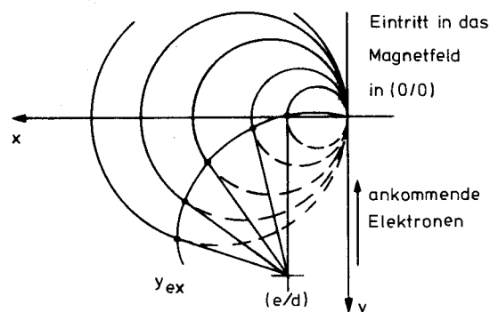
Fig.7 Polschuhkrümmung eines nichtdispersiven Magneten.
