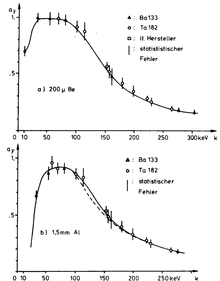
Fig.11 Ansprechwahrscheinlichkeit des Photonendetektors. Für die Messungen an C und Cu wurden Energien unterhalb 50keV nicht benötigt (1,5mm Al-Filter in b). In a) liegt bei 11keV die K-Kante von Germanium. In b) ist die Ansprechwahrscheinlichkeit, die sich mit der en-Bremsstrahlung an C als Referenz (s.u.) ergäbe, gestrichelt gezeichnet.
