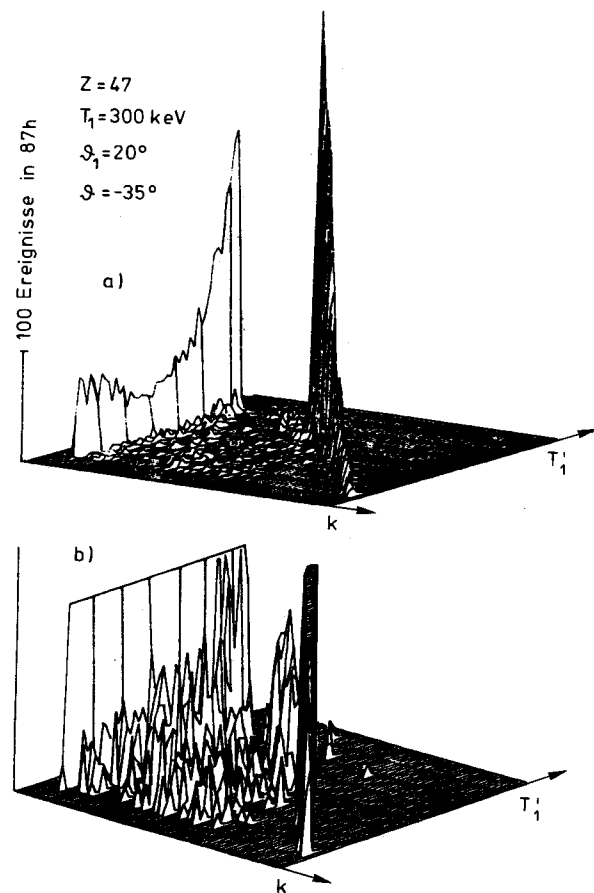
Fig.16 Differenzspektrum der Messung an Ag. Außer der diagonal verlaufenden en-Bremsstrahlung erscheint bei der Energie des in Koinzidenz nachgewiesenen charakteristischen Quants die Ionisation der K-Schale. Der Peak neben der en-Bremsstrahlung hat in der normierten Darstellung b) etwa die gleiche Höhe wie bei den Messungen an C und Cu: er kann der ee-Bremsstrahlung an den 45 äußeren Elektronen zugeordnet werden.
