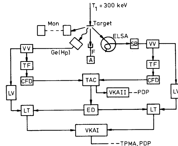
Fig.6 2p-Koinzidenzschaltung. Mon: Monitor, F/A: Faraday-Becher/Ampèremeter, Ge (Hp): Germaniumdetektor, ELSA: nichtdispersiver Magnet, SB: Oberflächensperrschichtzähler, VV: Vorverstärker, TF: Timing-Filter, CFD: Constant-Fraction-Discriminator, TAC: Zeit-Impulshöhen-Konverter, LV: Linearer Verstärker, LT: Lineares Tor, ED: Einkanal-Diskriminator, VKAII: Vielkanalanalysator (1p), VKAI: (2p), TPMA: Interface zum Zwischenrechner PDP 11-05.
