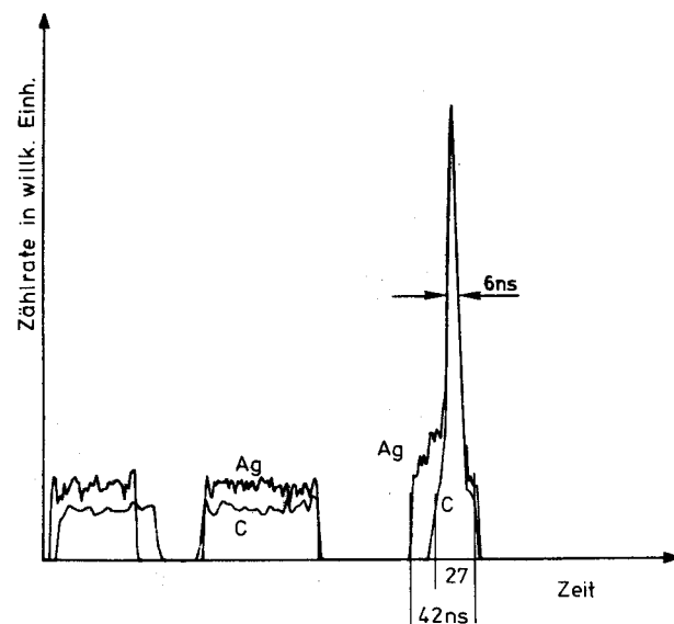
Fig.12 Zeitspektren einer Messung an Kohlenstoff und einer Messung an Silber. Die koinzidenten Ereignisse sind geroutet. Die Elektronenenergien liegen zwischen 40keV und 200keV, die Photonenenergien zwischen 15keV und 200keV (häufigste Energie jeweils ca. 150keV). Der Fuß des Ag-Peaks bei kleineren Zeiten entsteht durch das Wandern und die Verbreiterung der Koinzidenzlinie mit abnehmender Amplitude der Detektorsignale (bei der Messung an Ag sind niedere Energien häufiger vertreten).
