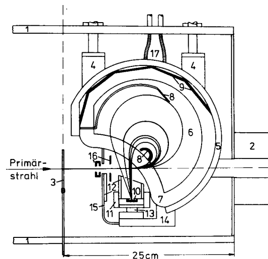
Fig. 10 Schnitt durch die Streukammer in der Symmetrieebene des Magneten. 1 Streukammer mit "Balkon" 2, in dem sich das Blendensystem mit Permanentmagneten für den Photonendetektor befindet. 3 Targethalter, 4 bewegliche Magnetaufhängung, 5 Joch, 6 Polschuh, 7 Spule in Polschuhform (quadratischer Querschnitt), 8 Energieblenden (C-Pb), 9 C-Platten, 10 Elektronendetektor, 11 Vorverstärker, 13 Peltierkühler, 14 Halterung (Cu-Ms), 15 C-Al-Pb-Abschirmung, 16 bewegliche Raumwinkelblenden (ohne Halterung), 17 Leitungen für Wasserkühlung. Bei den eingezeichneten Elektronenbahnen ist die räumliche Aufstreuung nicht berücksichtigt.
