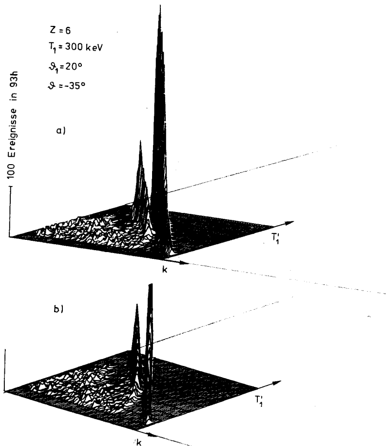
Fig.14 Differenzspektrum der Messung an C. In der Mitte der Ebene liegt von der en-Bremsstrahlung deutlich getrennt die ee-Bremsstrahlung mit ihrem gekrümmten Verlauf. Bei kleinen Energien liegt der durch die Compton-Streuung bzw. Elektronenrückstreuung verursachte Untergrund. Dabei verläuft die Compton-Kante entgegengesetzt gekrümmt zur ee-Bremsstrahlung und die "low-energetic-tails" liegen parallel zur T_1 -Achse.
