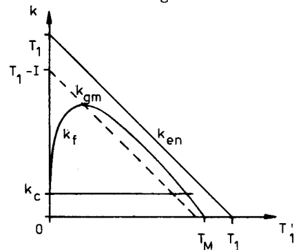
Fig. 4 Die Lage der inelastischen Prozesse in der T_1' - k -Ebene.
