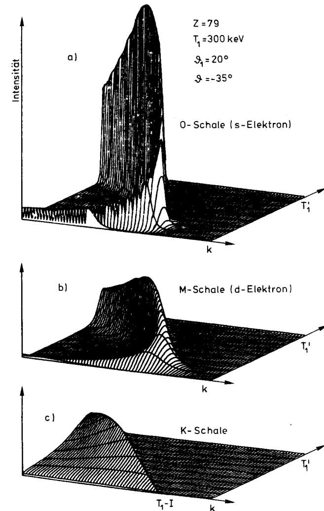
Fig.22 Zur Beeinflussung der ee-Bremsstrahlung durch die Bindung der Gold-Elektronen. a) O-Schale, 387eV, b) M-Schale, 5keV, c) K-Schale, 84keV. Jeweils ein Elektron.
