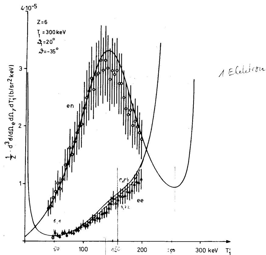
Fig.18 Wirkungsquerschnitte der en- und ee-Bremsstrahlung an Kohlenstoff. o: en, \Delta : ee. Theoretische Spektren nach (22) und (23). Gestrichelt: Berücksichtigung des Elwertfaktors für die ee-Bremsstrahlung. Meßparameter siehe Tab.1. Fehlerbalken: quadratisch gemittelter Gesamtfehler.
