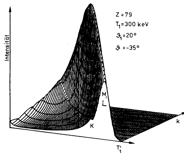
Fig.23 Mögliche Struktur der ee-Bremsstrahlung an Gold für alle Elektronen der K-, L- und M-Schale. Um das Spektrum der Ionisation der K-Schale ( k=0 ) sichtbar zu machen, liegt im Gegensatz zu Fig.22 hier die T_1' -Achse vorn.
