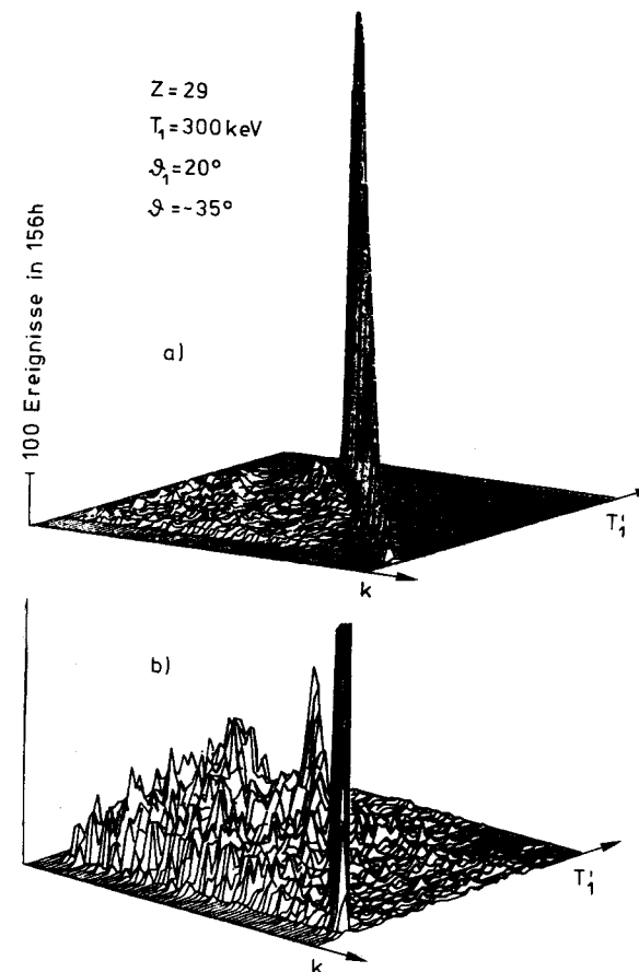
Fig.15 Differenzspektrum der Messung an Cu. Die ee-Bremsstrahlung ist in a) nur noch als kleine Erhebung neben der en-Bremsstrahlung zu erkennen. In der auf die Messung an C normierten Darstellung b) hebt sie sich jedoch bei großen Energien T_1 deutlich von der en-Bremsstrahlung und dem durch die Detektoren verursachten Untergrund ab.
