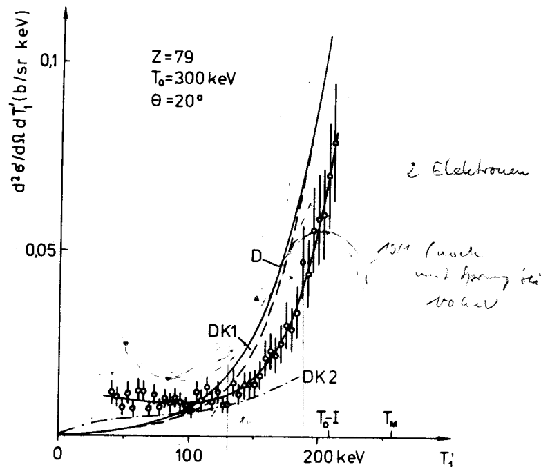
Fig.25 Zweifach differentieller Wirkungsquerschnitt der Ionisation der K-Schale von Gold in Abhängigkeit von der Energie des unter 20^\circ beobachteten Elektrons. Die Kurven "D", "DK1" und "DK2" sind im Text besprochen.
