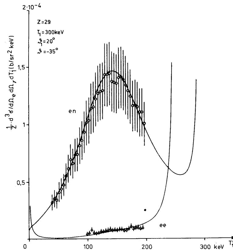
Fig.19 Wirkungsquerschnitte der en(o)- und ee( \Delta )-Bremsstrahlung an Kupfer. Meßparameter siehe Tab.1. Fehlerbalken: quadratisch gemittelter Gesamtfehler. Theoretische Spektren nach (22) und (23).
