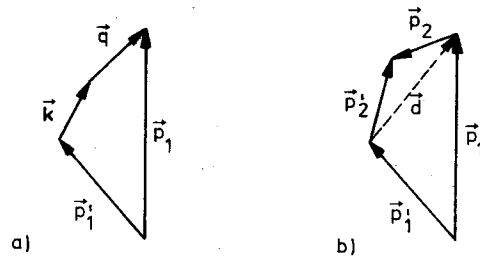
Fig. 2 Schematische Darstellung der Impulserhaltung bei der en-Bremsstrahlung (a) und der Ionisation (b). Die entstehenden Teilchen mit den Impulsen \vec{p}_1 und \vec{k} (a) bzw. \vec{p}_2 (b) können in beliebigen Richtungen beobachtet werden, da der Kern jeden Impuls \vec{q} aufnehmen kann, bzw. das Atomelektron jeden Impuls \vec{p}_2 liefern kann. Es ist zweckmäßig, den Impulsübertrag \vec{d} = \vec{p}_1 - \vec{p}_1' einzuführen. (das bei der Ionisation entstehende charakteristische Quant, das die Beobachtung dieses Prozesses ermöglicht, ist nicht eingezeichnet.)
