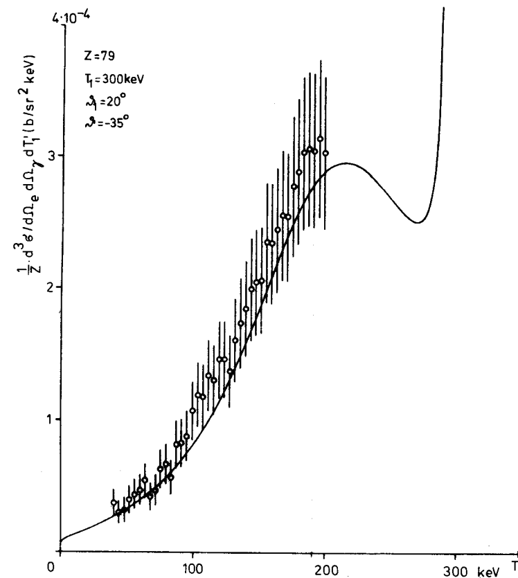
Fig.21 Wirkungsquerschnitt der en-Bremsstrahlung an Gold. Meßparameter siehe Tab.1. Fehlerbalken: quadratisch gemittelter Gesamtfehler. Theoretisches Spektrum nach (22), Abschirmung berücksichtigt.
