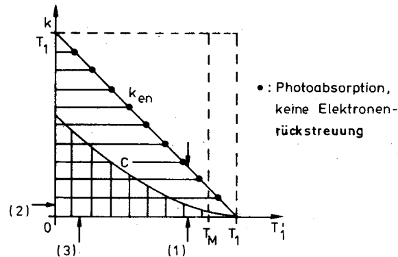
Fig.5 Durch echte Koinzidenzen der en-Bremsstrahlung und die Zählercharakteristiken hervorgerufener Untergrund. Wird die Teilchenenergie in den Halbleiterzählern nicht vollständig absorbiert, so entsteht in der T_1 -Richtung ein „low energetic tail“, in der k-Richtung das mit einer Kante (C) beginnende Compton Kontinuum. Die Pfeile deuten die zu erwartenden Grenzen des Meßbereiches an: starkes Anwachsen der zufälligen Koinzidenzen (1, 2) und mangelhafte Zeitauflösung (2, 3).
