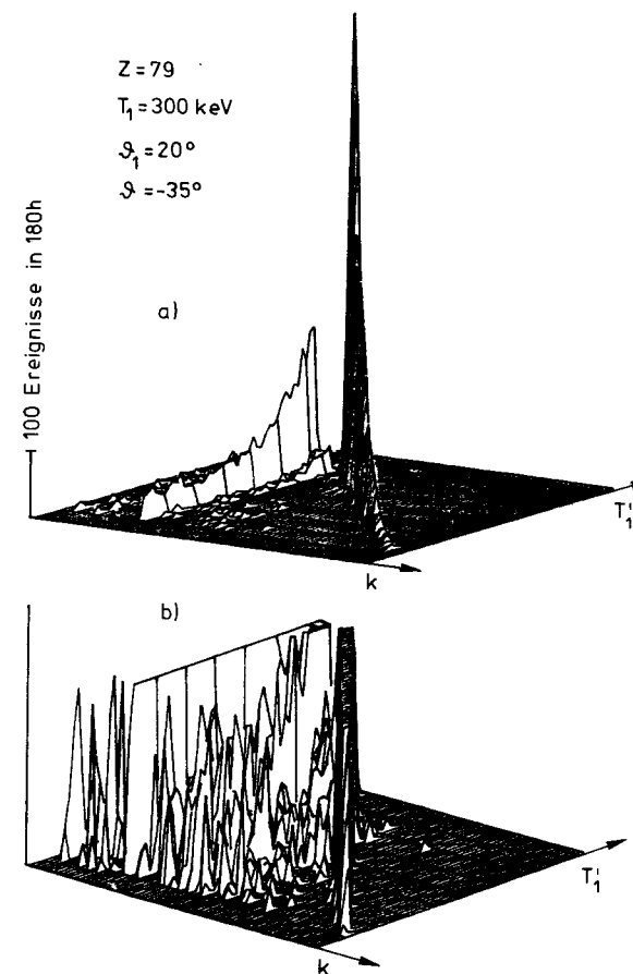
Fig.17 Differenzspektrum der Messung an Au. Im Vergleich zu der Messung an Ag wird in a) noch die Serienstruktur der K-Linie sichtbar. Vergleicht man die normierten Darstellungen b) der Messungen an den vier Elementen, so kann man vermuten, daß auch bei Au der neben der en-Bremsstrahlung liegende Peak durch die ee-Bremsstrahlung verursacht wird.
