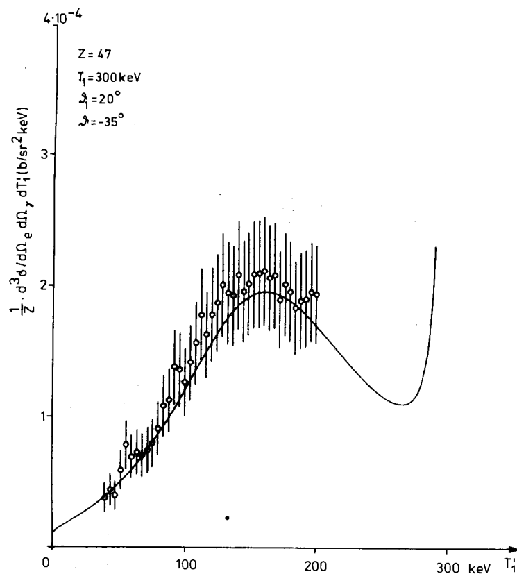
Fig.20 Wirkungsquerschnitt der en-Bremsstrahlung an Silber. Meßparameter siehe Tab.1. Fehlerbalken: quadratisch gemittelter Gesamtfehler. Theoretisches Spektrum nach (22), Abschirmung berücksichtigt.
