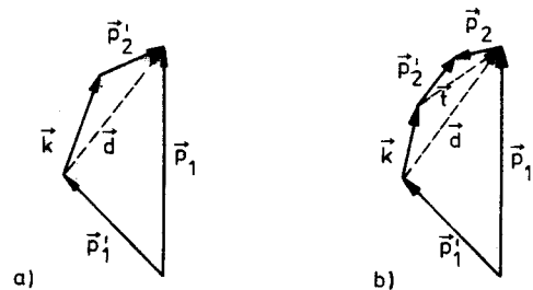
Fig. 3 Schematische Darstellung der Impulserhaltung bei der ee-Bremsstrahlung am freien (a) und am gebundenen (b) Elektron. Im Falle des freien Elektrons ist nach der Vorgabe von \vec{p}_1 und einer weiteren Richtung der Rest durch die Erhaltungssätze festgelegt. Durch den Impuls \vec{p}_2 des Atomelektrons wird wie in Fig. 2 diese Abhängigkeit aufgehoben. Außer durch \vec{d} ist durch \vec{t} in b) eine weitere Symmetrieachse gegeben.
