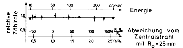
Fig.8 Abhängigkeit der Elektronenzähne von der Energie.
